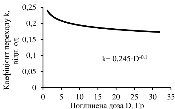
Рис. 2. Залежність коефіцієнта переходу 131 I у ЩЗ від поглиненої в органі дози.
