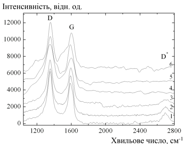
Рис. 3. Спектри КРС, отримані для БВНТ у вихідному (неопромінену) стані (1) і після електронного опромінення при дозах поглинання 3,0 (2), 4,0 (3), 6,0 (4), 8,0 (5) і 10,0 (6) МГр ( \lambda_{\text{вб}} = 514,5 нм, E_e = 1,8 MeV).
