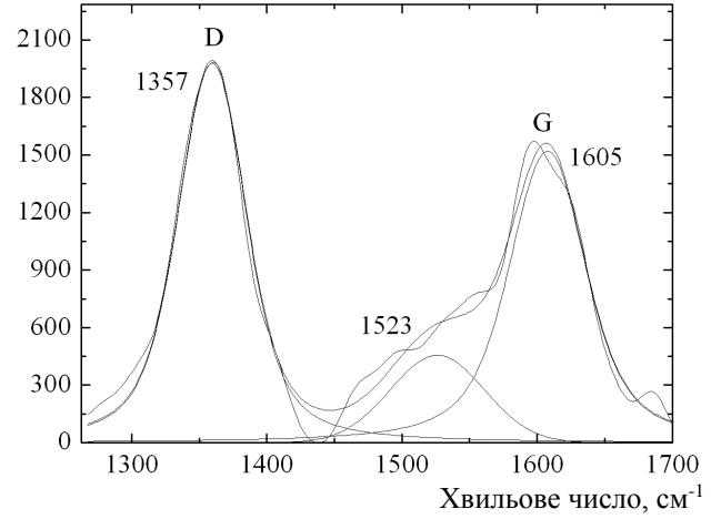
Рис. 4. Компоненти смуг D і G спектра КРС для БВНТ після електронного опромінення з дозами поглинання 8,0 ( a ) і 10,0 МГр ( б ).
