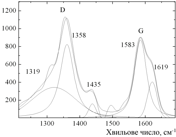
Рис. 4. Компоненти смуг D і G спектра КРС для БВНТ після електронного опромінення з дозами поглинання 8,0 ( a ) і 10,0 МГр ( б ).
