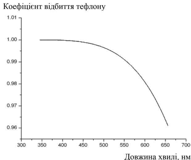
Рис. 4. Крива спектральної залежності коефіцієнта відбивання тефлонової плівки від довжини хвилі.
