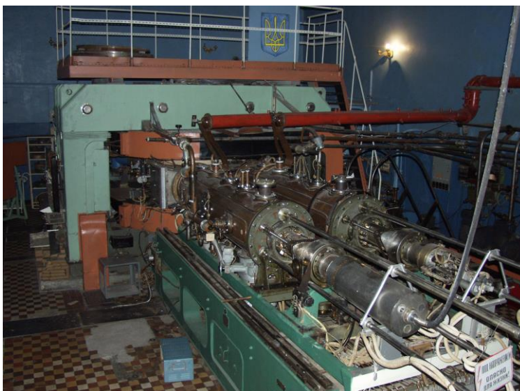
Циклотрон У-120.
