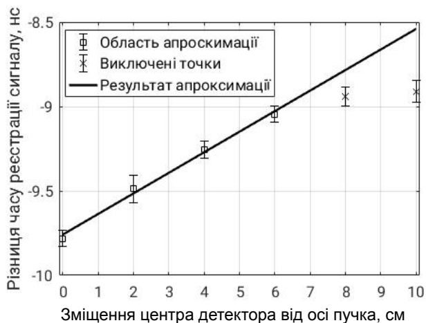
Рис. 5. Залежність різниці часу реєстрації сигналу на кінцях кварцового детектора залежно від його зміщення відносно центра пучка.
