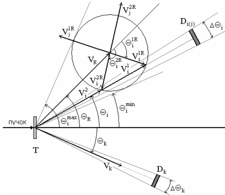
Рис. 3. Векторна діаграма швидкостей для реакції p + T \rightarrow k + i + j . \Theta_k, \Theta_i, \Theta_R , V_k, V_i, V_R – кути емісії та швидкості в л.с.к. частинок k, i та центра інерції резонансу R відповідно. D_k, D_{i(j)} – детектори, що реєструють частинки k та i . Радіус кола відповідає можливим значенням V_i^R (швидкості частинки i в системі центра мас ядра R ).
