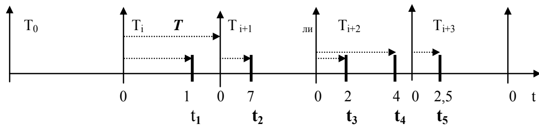
Рис. 4. Временная диаграммы регистрации данных.
