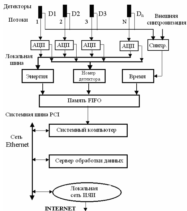
Рис. 1. Функциональная схема.
