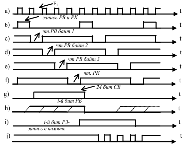
Рис. 6. Временная диаграмма работы.
